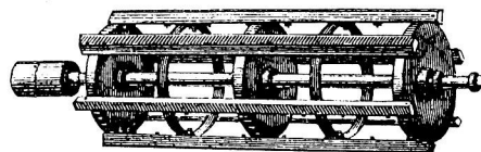
6. Trommel eener dorschmachine met slaglijsten
