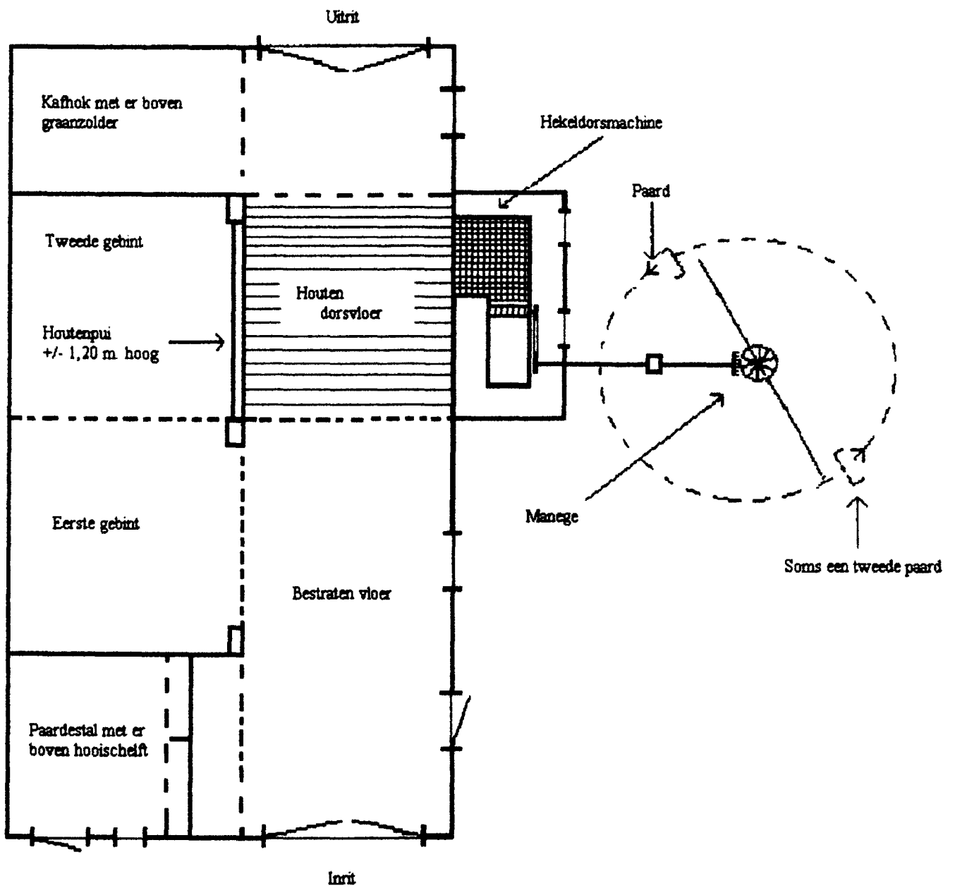
Indeling graanschuur met hekeldorsmachine
