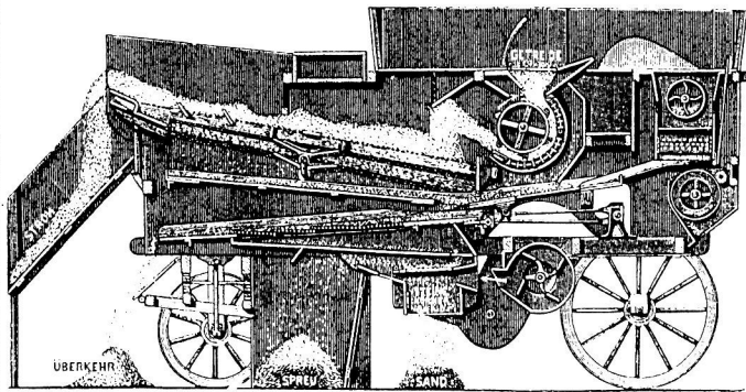
3. Overlangsche doorsnede eener stoom - dorschmachine.
