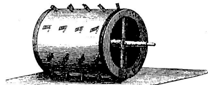
5. Hekeltrommel eener dorschmachine.
