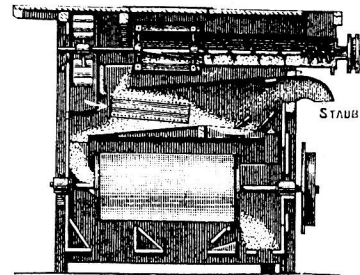
4. Dwarse doorsnede eener stoom - dorschmachine.
