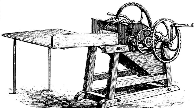
7. Handdorschmachine.
