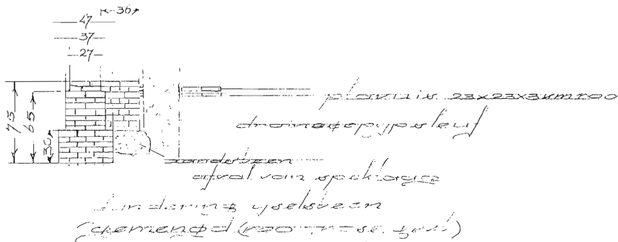
Doorsnede fundering en schouwvoet.
