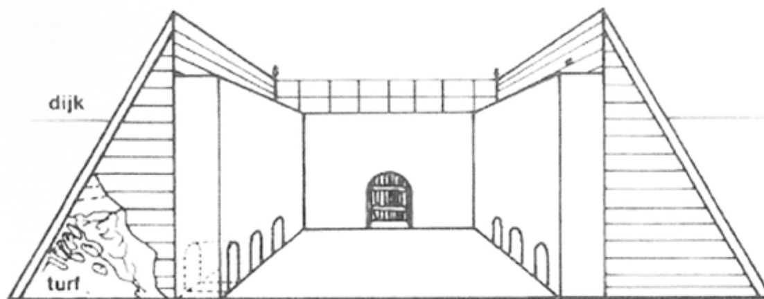
Schematische tekening van een veldoven. (internet)
