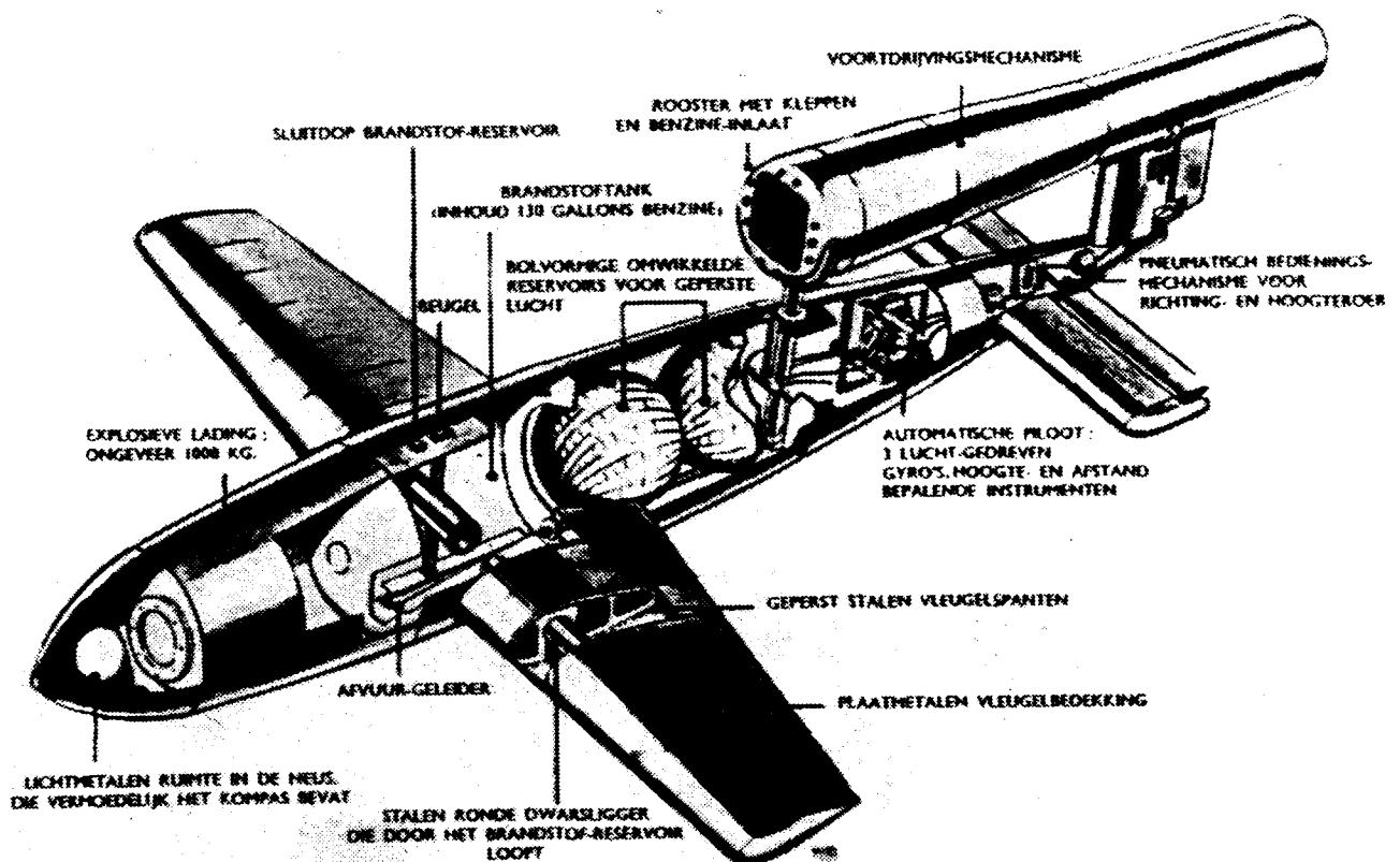
Doorsnede van een V-1.
